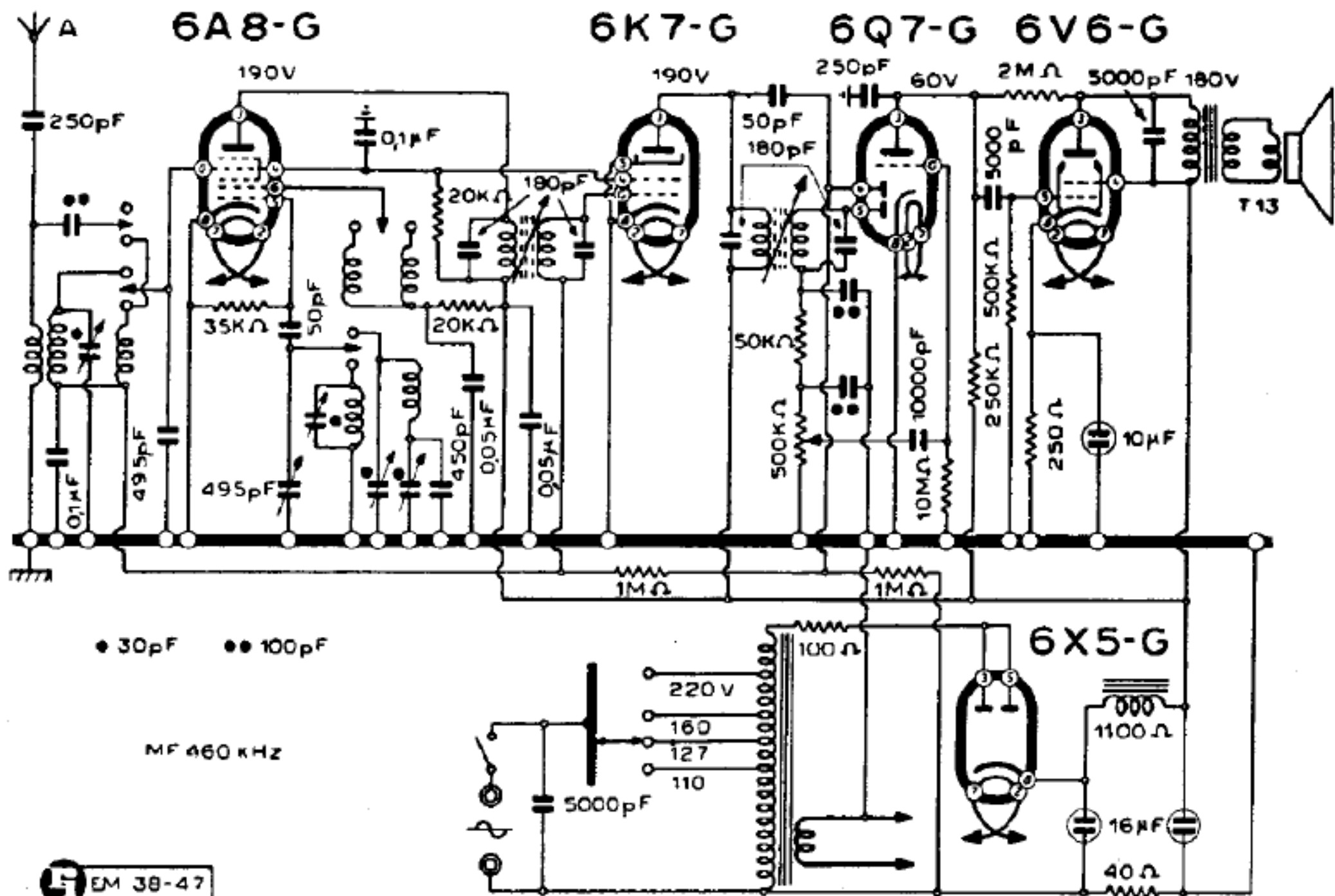
WATT RADIO - MOD. «AUREA PICCOLO 1948»
